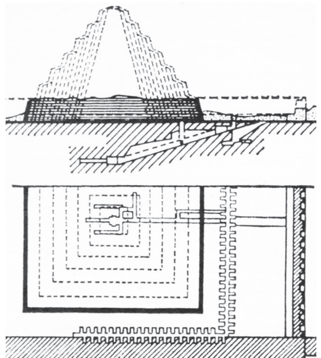
Пирамида Сехемхета в Саккара. Наверху разрез сохранившейся и незаконченной части; внизу горизонтальная проекция с подземными коридорами и камерами (по Гонейму)
