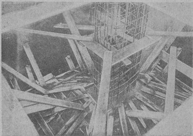
„Башмак“ — утолщенный конец фундаментной опоры главного здания. На рисунке — залитый бетонный башмак, с которого еще не снята опалубка. Видна арматура вертикальной колонны, еще не одетой опалубкой.
