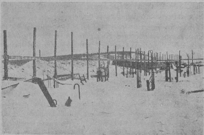
Законченные работы по устройству фундаментов главного здания в декабре 1930 г. На рисунке виден тепляк, в котором еще продолжают работы.
