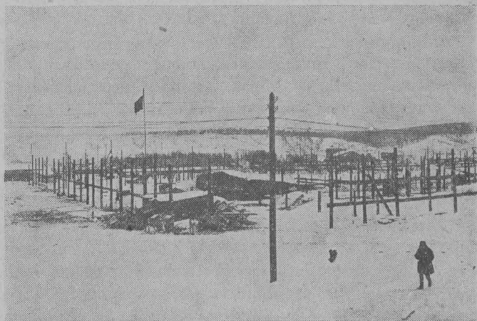
Вид работ по устройству фундаментных опор главного здания в январе 1931 г. В центре тепляк, в котором выдерживаются в тепле до полного отвердения (схватывания) железобетонные башмаки.
