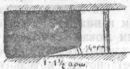
Рис. 13. Как производится подбойка или вруб, т. е. узкая щель, с ровердения которой начинается выемка угля.
