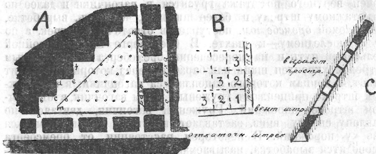
Рис. 14. Потолкоуступная система разработок.
