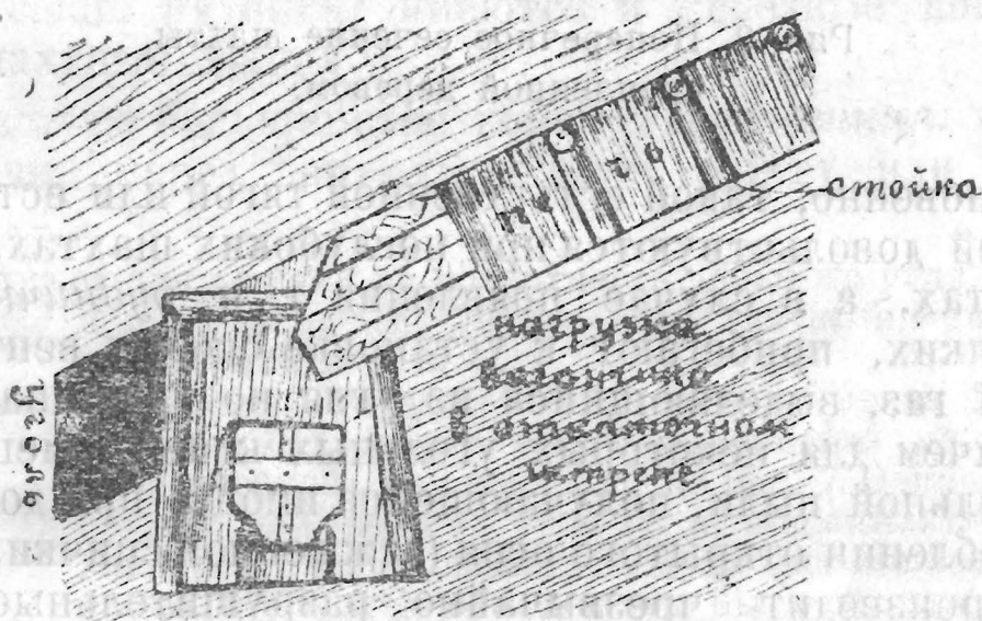
Рис. 10. Нагрузка вагончика в откаточном штреке, из печи уголь через деревянный люг сыпается в вагончик, стоящий на рельсах в откаточном штреке.
