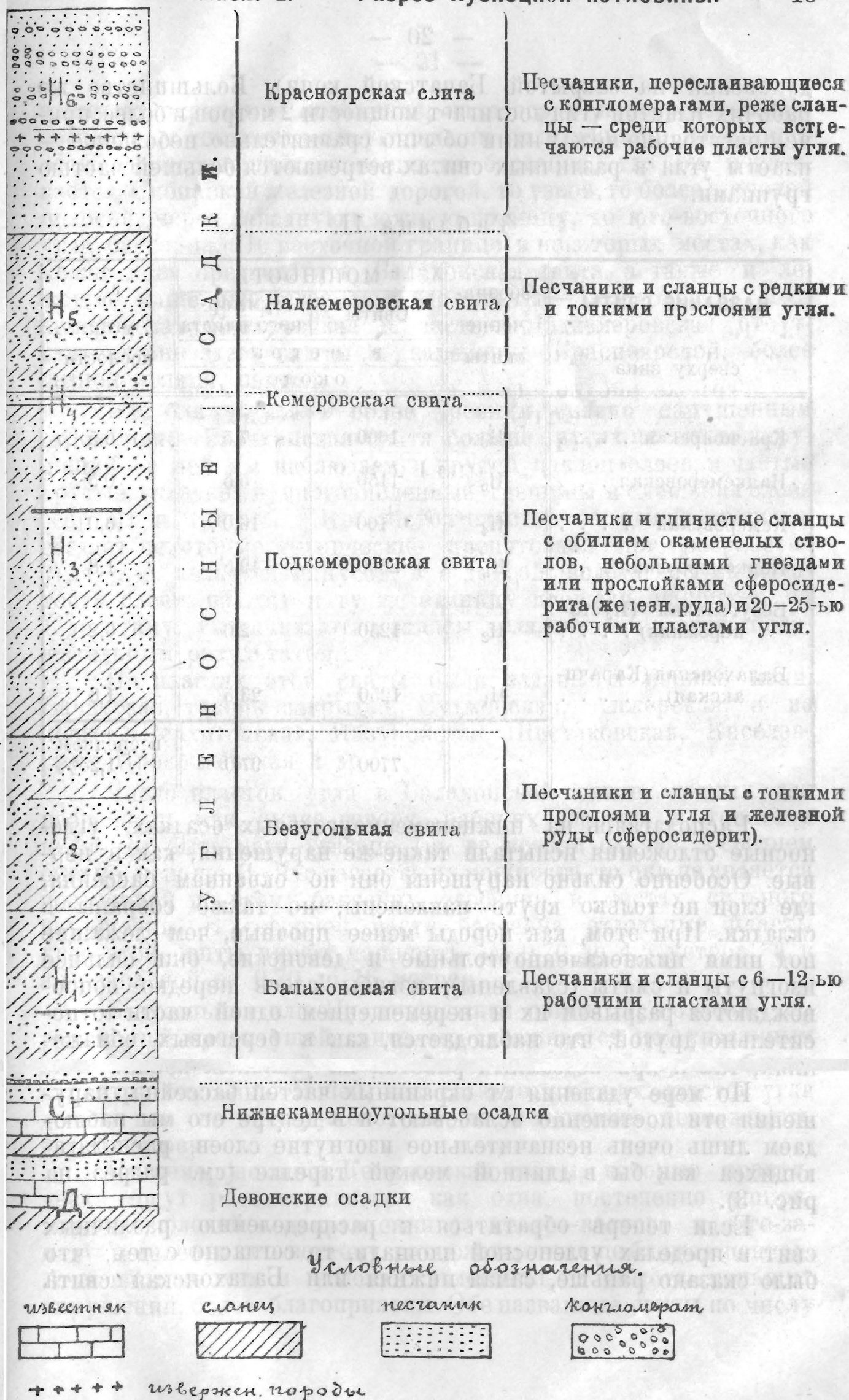
Рис. 5. Схематическая толща (легенда) осадков Кузнецкой котловины.
