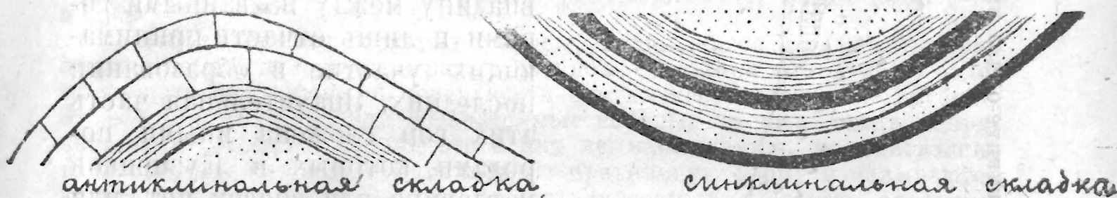
Рис. 2. Типы складок.
