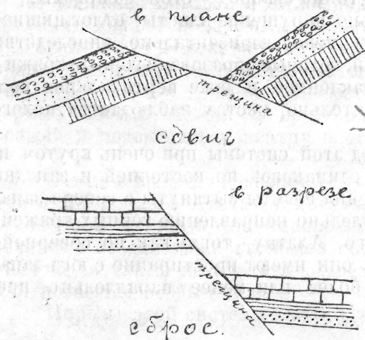
Рис. 4. Неправильности в залегании пластов.
