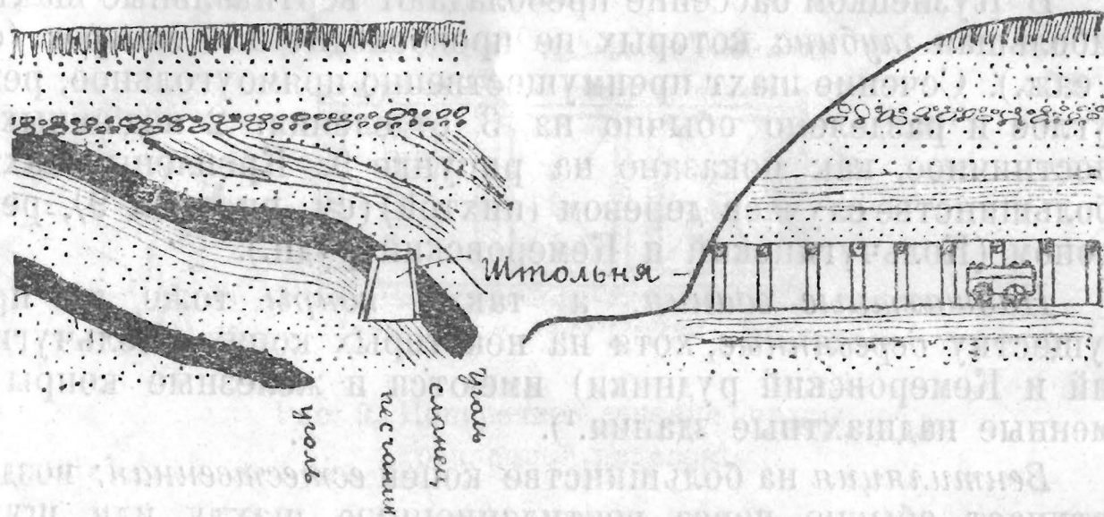
Рис. 6. Разработка полезного ископаемого (угля) штольней.
