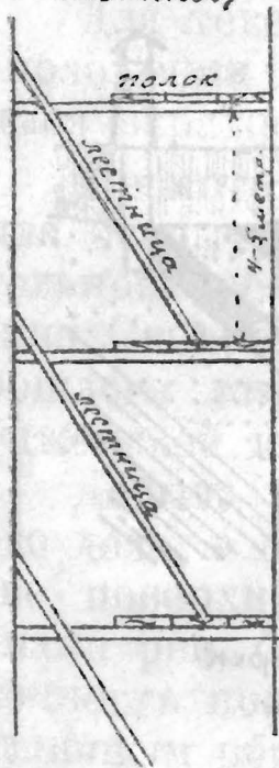
Рис. 8. Установка лестниц — вертикальный разрез по лестничному отделению шахты.
