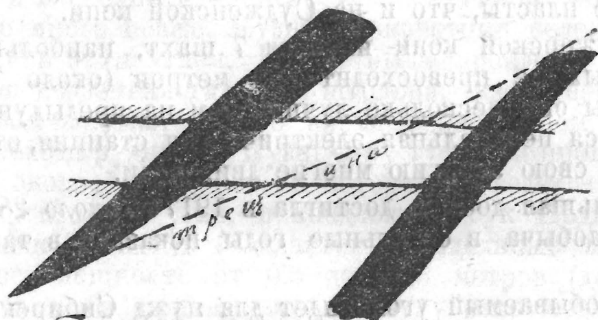
Пласт А повторился вследствие перемещ. части его по трещ.
