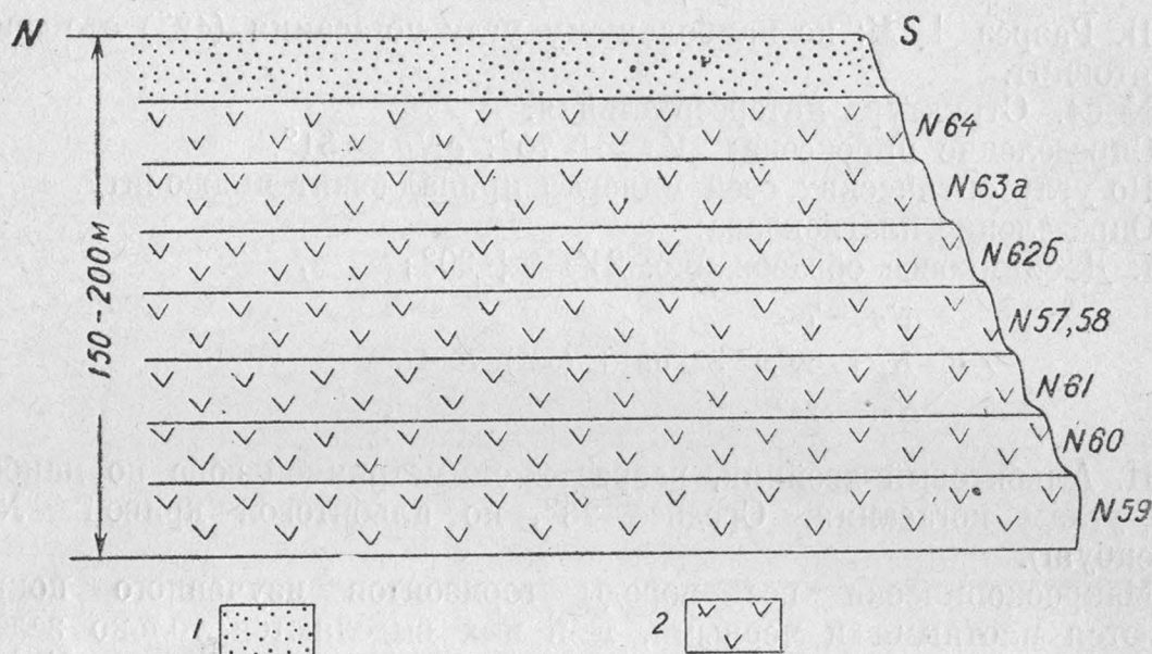
1 — песчаники; 2 — базальт.
