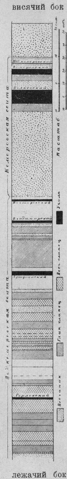
Рис. 4. Стопка угленосной толщи Кемеровской копи.
