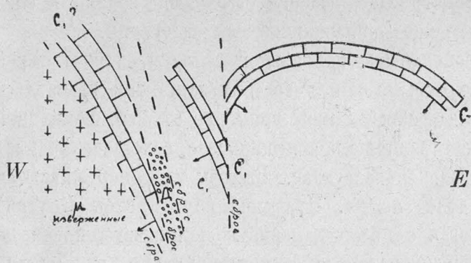
Рис. 1. Схема тектонических нарушений н. карбона в плане по р. М. Осиповой.
