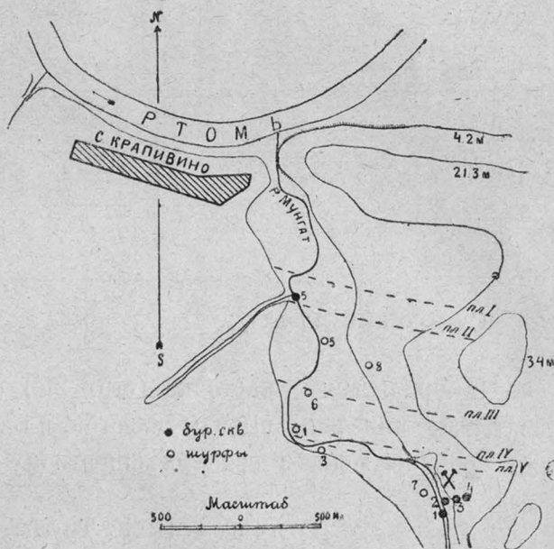
Рис. 5. План расположения шурфов и буровых скважин на Крапивинской копи.
