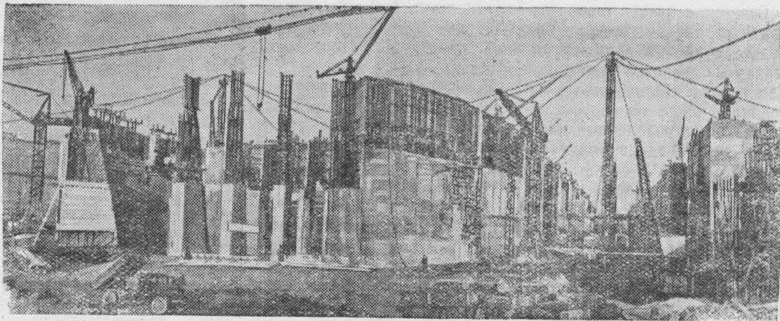
Куйбышевгидрострой. Первый пусковой объект Куйбышевского гидроузла—нижние судоходные шлюзы—вступит в строй весной этого года. День и ночь на громадной территории шлюзов кипит работа. Ведется укладка бетона на самых верхних ярусах, монтируется арматура, устанавливаются основные механизмы управления.
