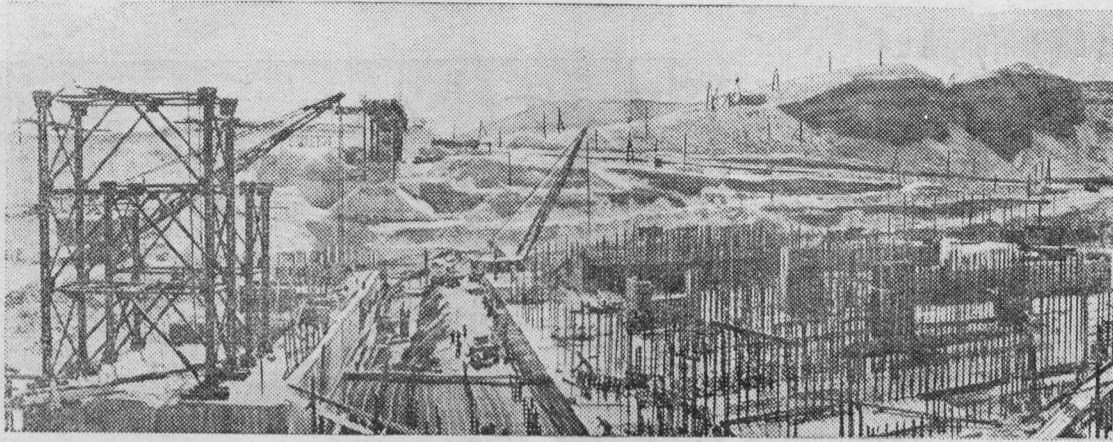
В Таджикистане, близ Ленинабада, на реке Сур-Дарье строится крупнейшая в Средней Азии Кайраккумская гидроэлектростанция. На снимке: общий вид строительства водосливной плотины и здания Кайраккумской гидроэлектростанции.
