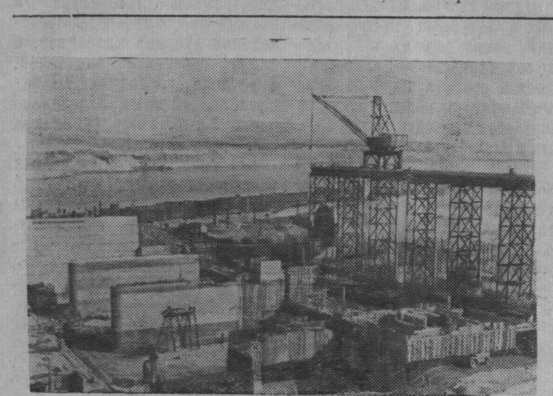
Таджикская ССР. Недалеко от Ленинабада, в урочище Кайрак-кум, сооружается самая крупная в Средней Азии гидроэлектростанция, которая даст ток многим промышленным предприятиям, городам, поселкам, школам Таджикистана и Узбекистана. Страна обеспечила стройку на Сыр-Дарье новейшей техникой и высококвалифицированными кадрами строителей. Пуск первого агрегата гидроэлектростанции намечен осенью 1956 года. Строители развешивают соревнования в честь XX съезда КПСС и настойчиво добиваются сокращения сроков работ.
