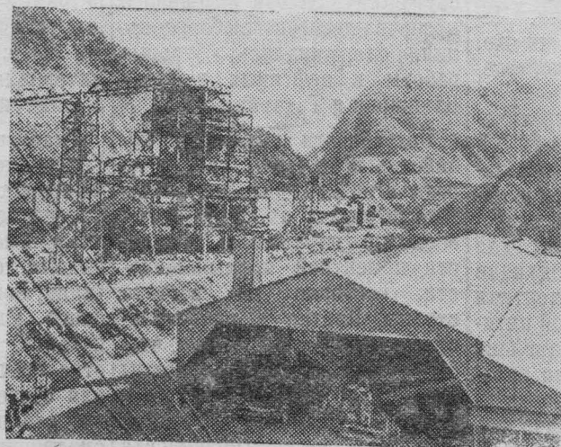
Индия. В живописных ущельях отрогов Гималаев развернулось строительство плотин и электростанций Бхакра-Нангал. НА СНИМКЕ: один из участников сооружения плотины. Слева—бетонный завод.
