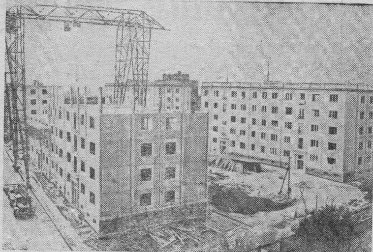
В Чехословацкой Республике внедряется метод строительства домов из готовых панелей. После успешных опытов в г. Готвальдове (Моравия) сейчас ведется сооружение из панелей шести 40-квартирных домов в одном из районов чехословацкой столицы Праги. Части стен или целую стену комнаты укладывают при помощи больших подъемных кранов.
