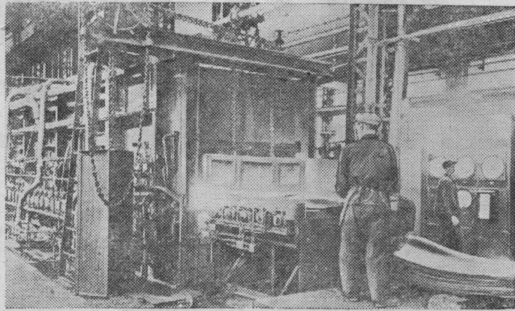
Москва. Металлурги завода «Серп и молот» готовят достойную встречу XX съезду КПСС. На предприятии внедряется новая техника, совершенствуется технология. На мартеновских печах внедрены термостойкие своды, комплексная автоматика, используется кислород для ускорения выплавки металла. В листопрокатном цехе пущена новая высокопроизводительная роликовая печь. По сравнению с прежней печью производительность ее в два раза больше. НА СНИМКЕ: новая роликовая печь в листопрокатном цехе завода.
