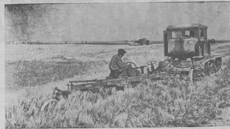
Белорусская ССР. В колхозе имени Гастелло выделен опытный участок, который обрабатывается по методу Т. С. Мальцева. Для этой цели механизаторы Минской МТС сняли у пятикорпусного плуга «П5-35» отвалы и предплужники, отрегулировали плуг для вспашки на глубину 40—45 сантиметров.
