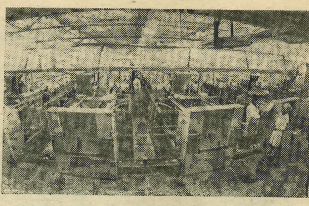
птицеводом-оператором на главном пульте управления цеха-автомата; один из блоков цеха-автомата, где одновременно содержится 140 тысяч кур.
