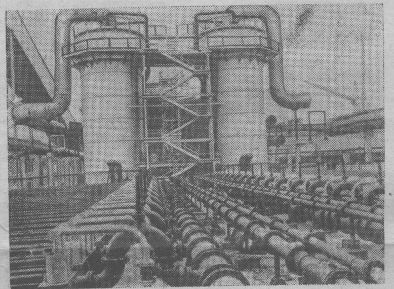
Комбинат сложных минеральных удобрений в Девне — крупнейшая новостройка Болгарии. Этот центр большой химии спроектирован софийским научно-исследовательским институтом «Химпроект» при содействии советских специалистов. Все производственные процессы на нем механизированы и автоматизированы и управляются при помощи электронно-вычислительной техники.
