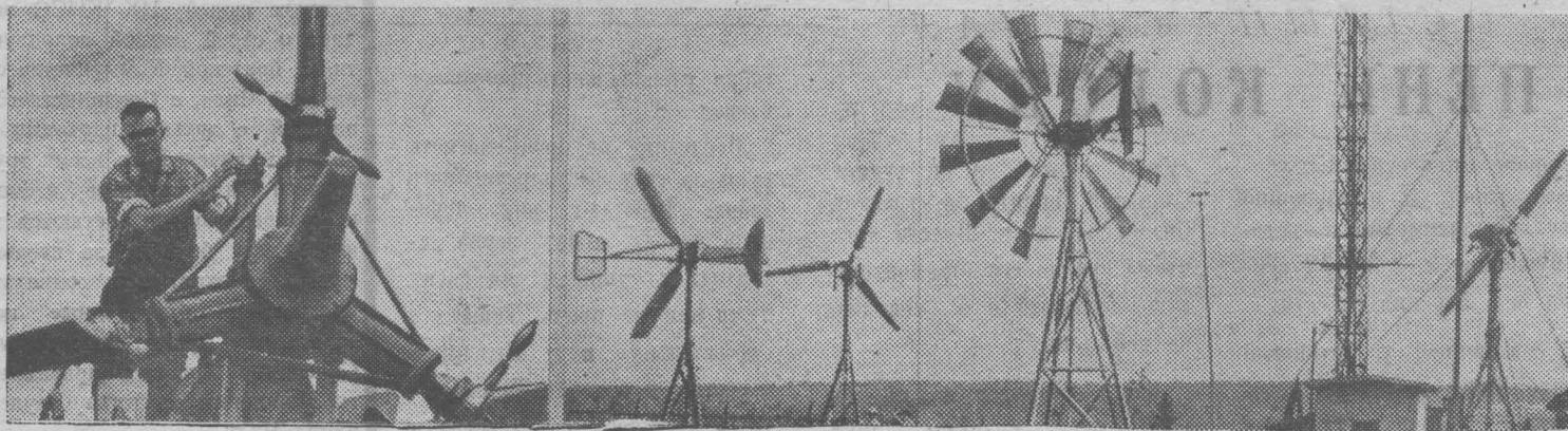
МОСКОВСКАЯ ОБЛАСТЬ. В Истринском районе расположен единственный в нашей стране и мире испытательный полигон ветроустановок Всесоюзного института электрификации сельского хозяйства. На полигоне сейчас проходят проверку несколько агрегатов, созданных в лаборатории эксплуатации и ветроэнергетических установок, которой руководит доктор технических наук Я. И. Шехтер. Созданию ветровых установок уделяют большое внимание в ФРГ, Канаде, США и других государствах. Несколько десятков стран изъявили желание приобрести в Советском Союзе ветроустановки различного назначения, которые по праву считаются лучшими в мире. На снимках (слева): начальник полигона Г. Струков на монтаже ветроустановки «Сокол». За один час она может поднять 15 кубометров воды с глубины 110 метров; панорама ветрополигона.
