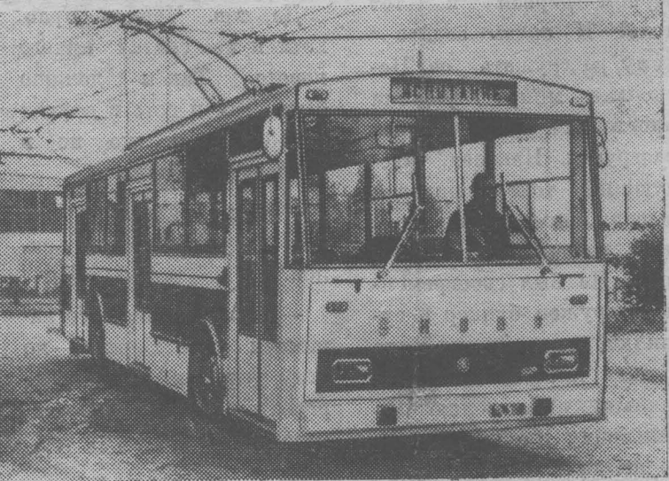
ЧССР. Жители двадцати пяти советских городов ездят в удобных и быстрых троллейбусах, построенных руками мастеров завода «Шкода» в западно-чешском городе Остров. Только в нынешнем году Советский Союз получит 400 современных троллейбусов. На снимке: заводские испытания проходит троллейбус «Т-14», который более быстроходен, комфортабелен и экономичен, чем его предшественники. Фото ЧТК—ТАСС
