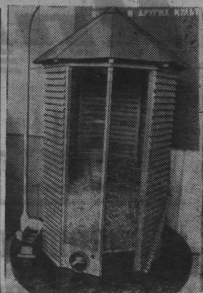
МОСКВА. На Выставке достижений народного хозяйства СССР демонстрируется макет нового механизированного сенокосилки башенного типа, снабженного системой досушивания сена во время хранения способом вентилирования. Хранилище вмещает 100 тонн сена и оборудовано устройствами механической погрузки и выгрузки.
