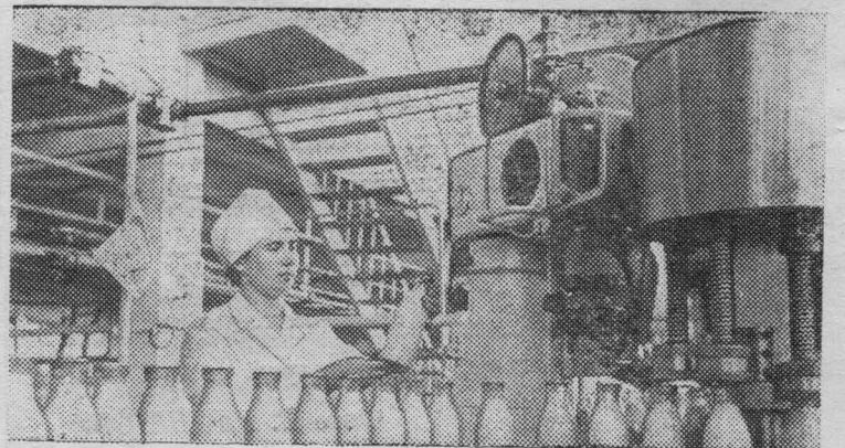
В Чернигове сдана в эксплуатацию первая очередь нового молокозавода с проектной мощностью 100 тонн молочных продуктов в смену. Предприятие оснащено новейшей отечественной аппаратурой.
