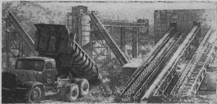
В Амурской области на берегах реки Зеи строится Зейская гидроэлектростанция. Это первенец гидроэнергетики на Дальнем Востоке. Мощность электростанции почти полтора миллиона киловатт.
