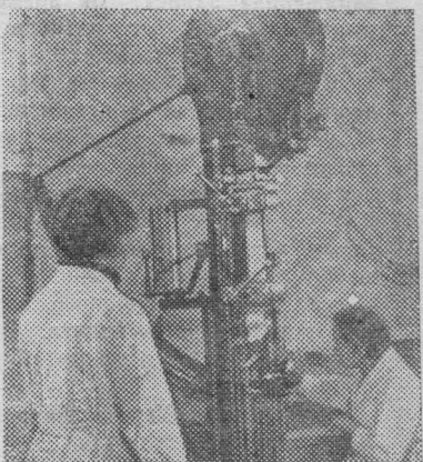
Испытание ткани на разрыв для парашюта спускаемого аппарата автоматической межпланетной станции «Венера-7».
