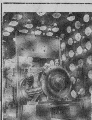
МОСКВА. В сентябре здесь откроется Международная выставка «Химия-70». Среди экспонатов посетители увидят автоматизированную аммиачную холодильную установку «УА-100», выпуск которой освоен заводом «Компрессор». Установка предназначена для различных отраслей народного хозяйства, в том числе, для предприятий, связанных с производством, хранением и переработкой сельскохозяйственной продукции.
