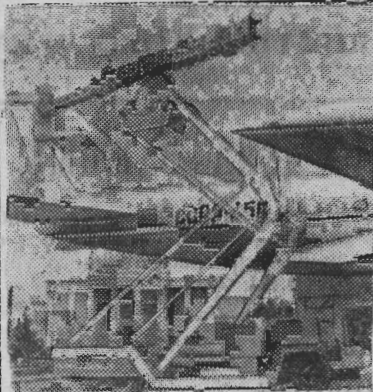
МОСКВА. Эта самоходная механизированная установка «МММ-1» для наружной мойки самолетов всех современных марок, появившаяся недавно на ВДНХ СССР, создана на одном из заводов Министерства гражданской авиации СССР.
