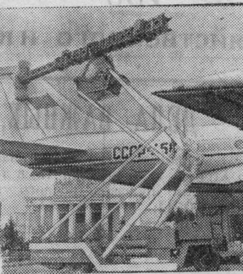
МОСКВА. Эта самоходная механизированная установка «МММ-1» для наружной мойки самолетов всех современных марок, появившаяся недавно на ВДНХ СССР, создана на одном из заводов Министерства гражданской авиации СССР.
