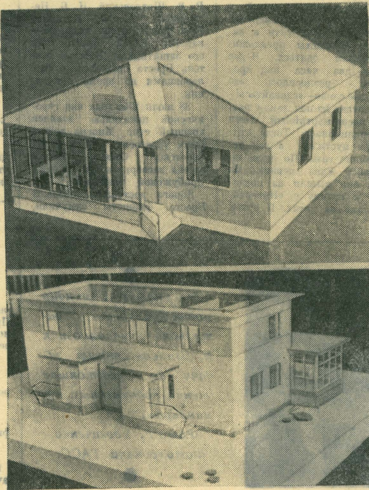
Экспериментальный проект жилого дома с 4-комнатными квартирами в двух уровнях со стенами из ячеистобетонных блоков. Фото Н. Акимов и А. Стужина.
