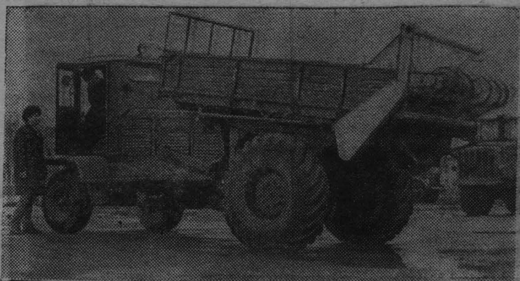
Запорожье. Разбрасыватель органических удобрений РНШ-4 создан коллективом конструкторского бюро Министерства тракторного и сельскохозяйственного машиностроения. Он обладает высокой проходимостью и маневренностью. Загрузка удобрений может осуществляться всеми видами погрузчиков. При попадании в кузов вместе с удобрениями посторонних предметов нормальная работа не нарушается.
