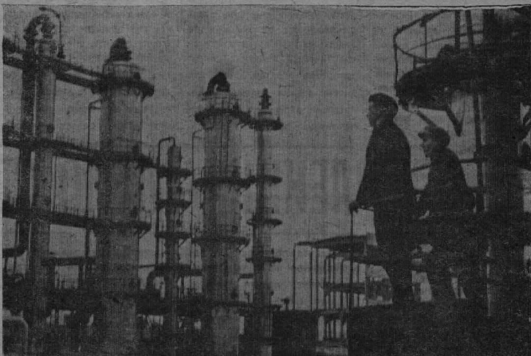
Ново-Кемеровский химкомбинат. Скоро вступит в строй очередь комплекса капролактама. Корпуса оснащены отечественным оборудованием и будут работать на более дешевом сырье.
