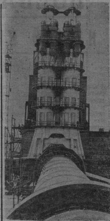
В Бернбурге (округ Галле) пущена в пробную эксплуата- цию первая в Германской Де- мократической Республике установка по выпуску цемент- ного клинкера сухим спосо- бом. Это высоко-автомати- зированное производство, от- вечающее требованиям миро- вых стандартов. Мощность— 1.200 тонн клинкера в день. Фото АДН—ТАСС.
