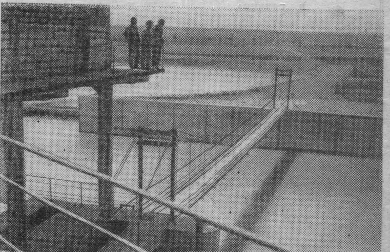
АРМЯНСКАЯ ССР. На строительстве крупнейшей в республике Мхчанской насосной станции идет прокладка и монтаж трехлинейного трубопровода, сооружаются дамбы на Севджурском головном участке и у Нижне-Разданского канала. С вводом станции в эксплуатацию свыше 20 тысяч гектаров земель Арташатского и Вединского районов в 1969 году получат воду. На снимке: сооружения Мхчанской насосной станции на Севджурском головном участке. Фото З. Исаакяна и Б. Немрута. Фотохроника ТАСС.
