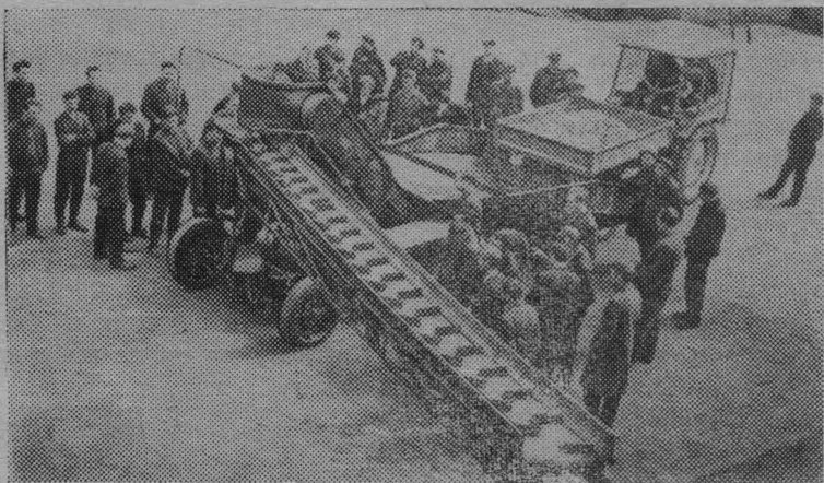
ЭСТОНСКАЯ ССР. Тартуский завод сельскохозяйственных машин «Вийт» приступил к изготовлению транспортеров-грузчиков ТЗК-30, работающих при помощи электроэнергии. Машины предназначены для погрузки картофеля, их производительность 30 тонн в час. В этом году завод изготовит 250 таких транспортеров.
