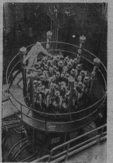
Реактор Нововоронежской атомной электростанции.
