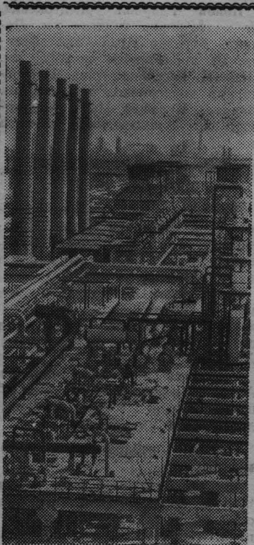
Азербайджанская ССР. 26 объектов комплекса этилена, первая очередь Сумгаитского химического комбината — Всесоюзной ударной комсомольско-молодежной стройки — накануне сдачи в эксплуатацию. В разгаре пусконаладочные работы. На снимке: комплекс этилена. Фото Ю. Рахила. Фотохроника ТАСС.
