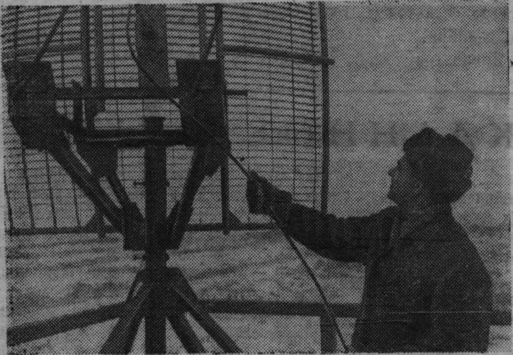
ЗАПОРОЖСКАЯ ОБЛАСТЬ. Этот снимок сделан на высоте 38 метров. Электромеханик Михайловской районной конторы связи В. Плющ проверяет направленную антенну. Недавно в районном центре Михайловке закончен монтаж новой радио-релейной линии, которая обеспечила связь района с Мелитополем и Днепродзудным.
