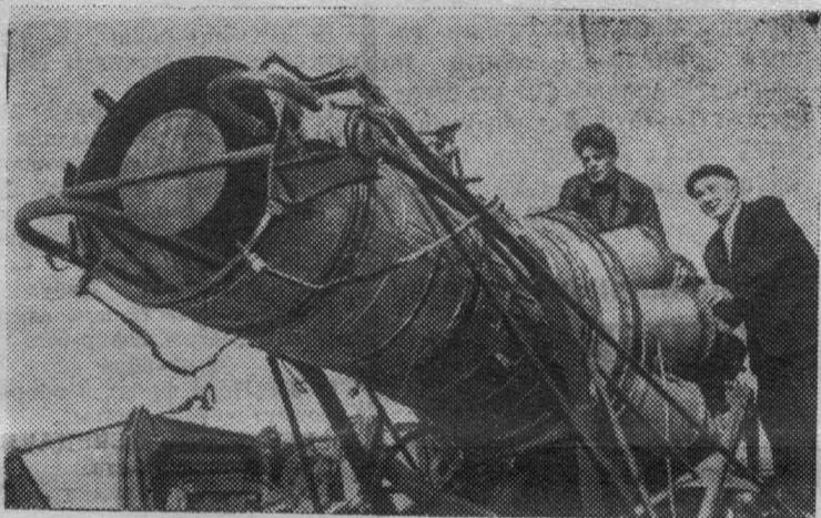
В Институте химической кинетики и горения Сибирского отделения Академии наук СССР разработан этот мощный аэрозольный генератор на базе турбореактивного двигателя, установка успешно используется в борьбе с гнусом и вредителями сельского хозяйства.
