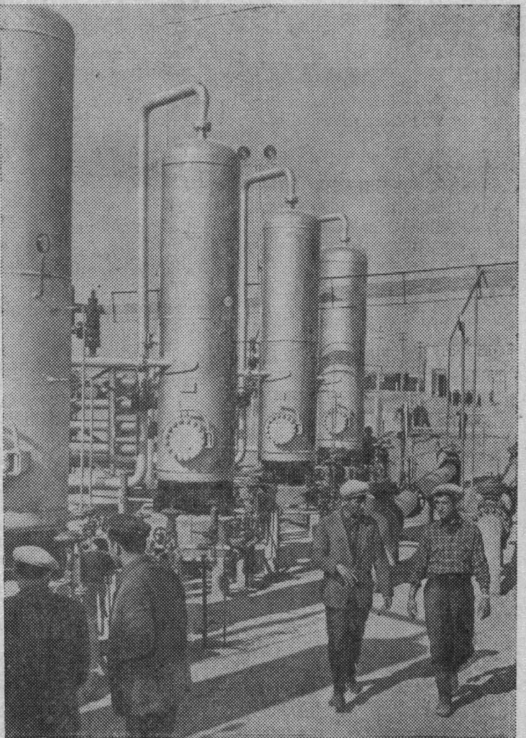
Газосборный пункт на Очакском месторождении. Фото К. Мурадова.
