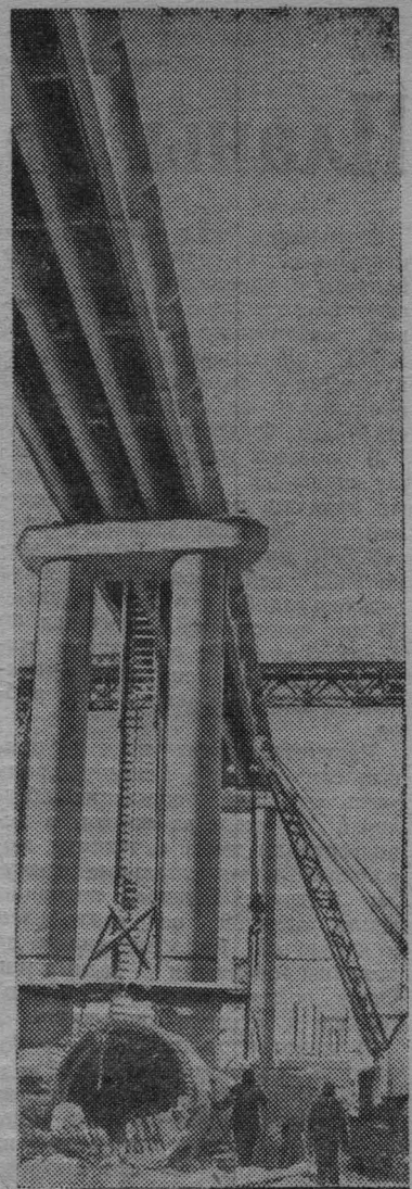
На снимках: сверху — строительство автомобильного моста через пролив Кивисиллансальми близ г. Выборга. Он сооружается советскими специалистами. Мост свяжет г. Выборг с Сайменским каналом. Слева — финские специалисты Р. Юрванен и С. Карху на трассе строительства шлюза в Юстала.
