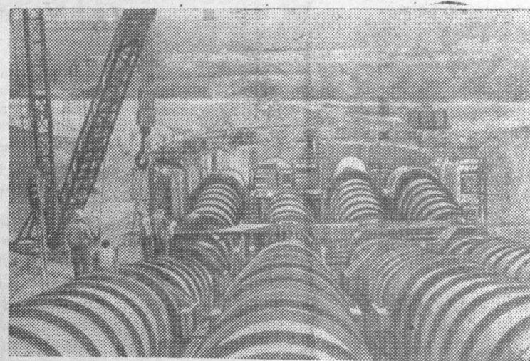
Почти третья часть полноноволного Иртыш будет поднята на высоту Эйфелевой башни и переброшена на 475 километров в Карагану с помощью двадцати двух насосных станций.
