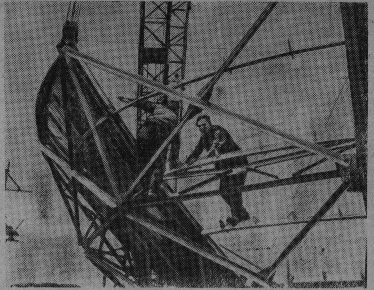
Монтаж мощного радиотелескопа на территории астрономической обсерватории Краковского университета (Польша). Диаметр антенны радиотелескопа — 12 метров. Фото ЦАФ — ТАСС.
