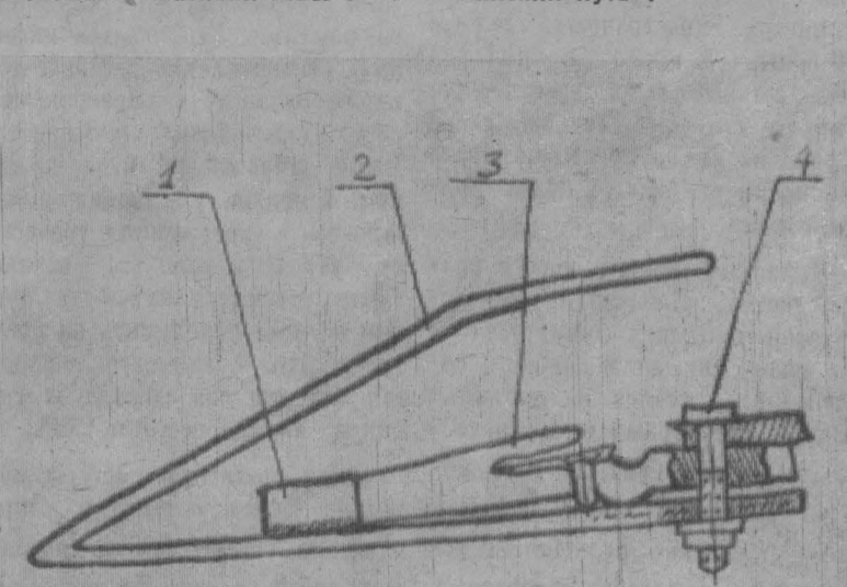
На рисунке: 1 — наконечник; 2 — стержень стеблеподъемника; 3 — палец режущего аппарата; 4 — болт.
