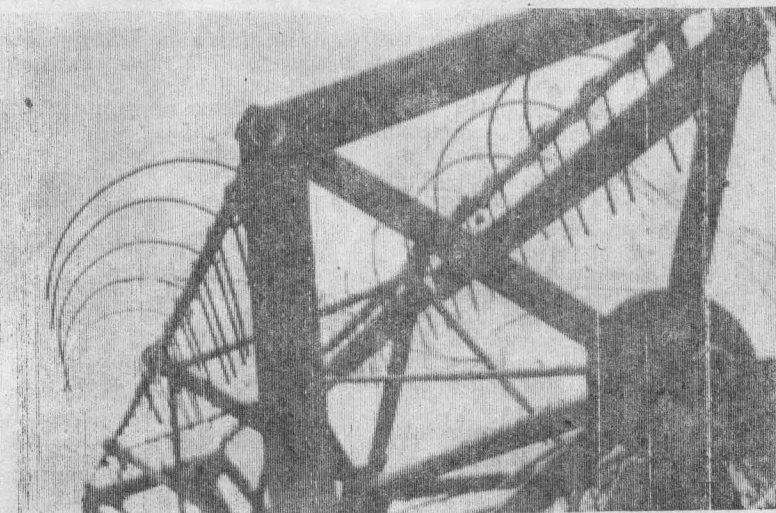
Так выглядит эксцентриковое мотопило жатки, оборудованное приспособлениями Морозова.
