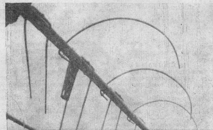
Крепление зубьев на трубе мотопилы осуществляется с помощью шплинтов. Фото И. ВАСЬКИНА.
