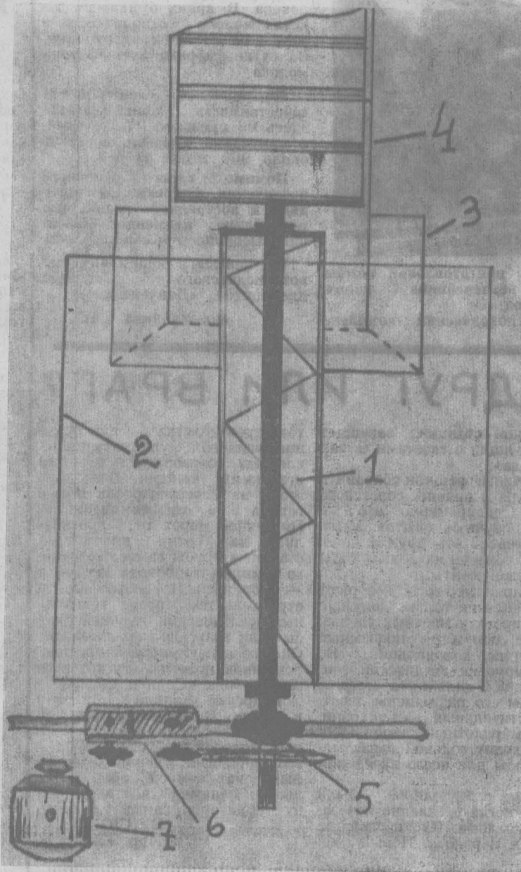
СХЕМА КОНСТРУКЦИИ КОРМОРАЗДАТЧИКА 1. Горизонтальный шнек бункера. 2. Бункер. 3. Приемный бункер горизонтального транспортера раздатчика. 4. Горизонтальный транспортер. 5. Корпуса подшипников. 6. Редуктор. 7. Электродвигатель.
