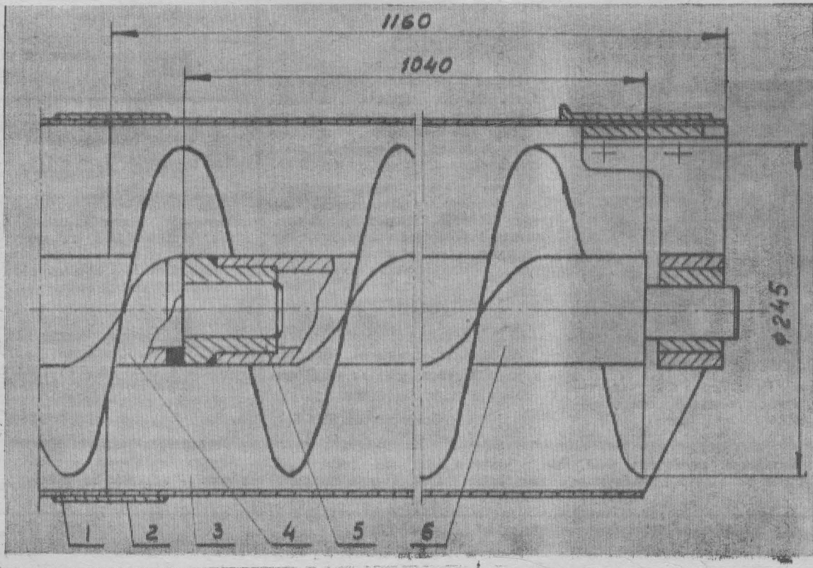
ЧЕРТЕЖ Б. (Размеры показаны в миллиметрах). Схема переходной втулки.
