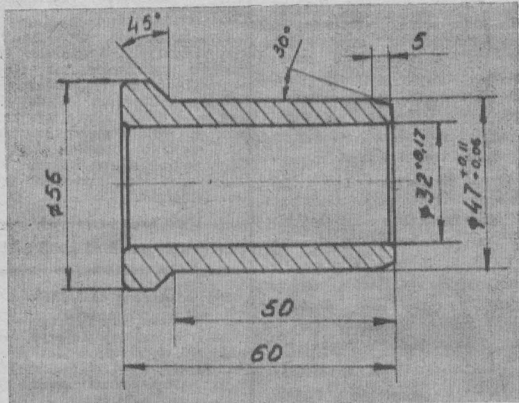
ЧЕРТЕЖ А. (Размеры показаны в миллиметрах). 1. Наращиваемая труба. 2. Соединительное кольцо. 3. Труба для наращивания. 4. Наращиваемый вал шнека. 5. Переходная втулка. 6. Вал для наращивания.
