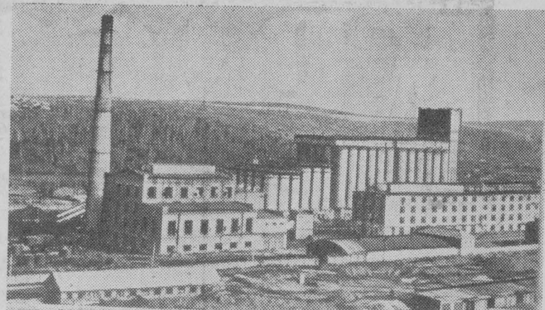
На окраине Иркутска, где еще недавно был пустырь, строится крупнейший в Сибири масложировой комбинат. В год он сможет перерабатывать на жиры и масло 163 тысячи тонн соевых и других семян.
