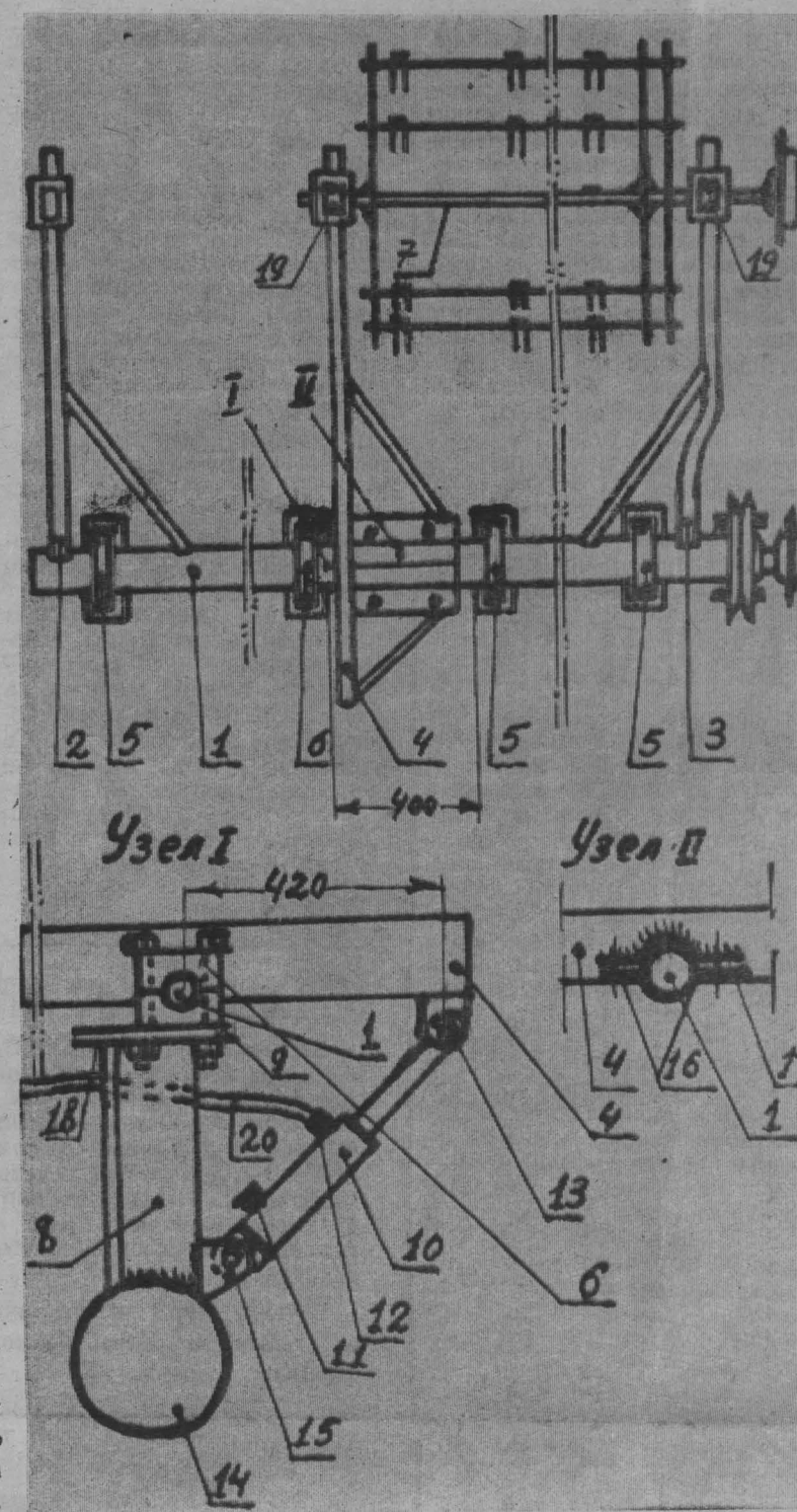
Схема переоборудования узлов жатки.
