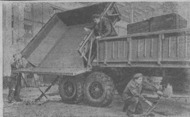
Коллектив Челябинского машиностроительного завода изготовил первую партию автотракторных прицепов 1-ПТС-9. Прицеп состоит из двух кузовов — переднего и заднего, грузоподъемность его — 9 тонн. Он может быть использован для перевозки зерна, кормов, строительных материалов, удобрений. С помощью специальной гидравлической установки, приводимой в действие от трактора, прицеп может разворачиваться на две стороны.
