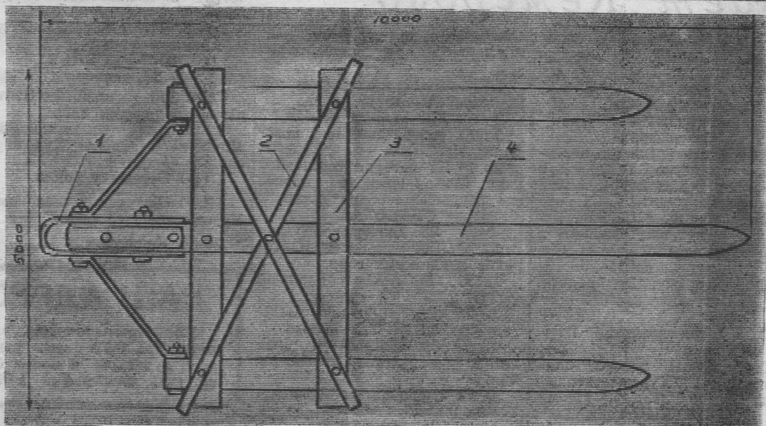
Волокуша-стоговоз. 1. Прицеп. 2. Растяжки. 3. Поперечный брус. 4. Полоз.
