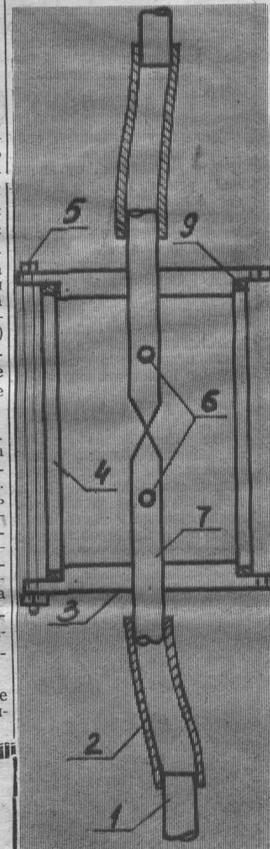
РИС. 2. ПРОДОЛЬНЫЙ РАЗРЕЗ ЭЛЕКТРОПОДОГРЕВАТЕЛЯ: 1. Водопроводная труба. 2. Резиновый шланг. 3. Металлический фланец. 4. Асбоцементная труба. 5. Стяжные болты. 6. Отверстия для холодной и горячей воды. 7. Труба подогревателя. 8. Резиновые прокладки.
