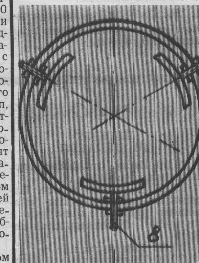
РИС. 3. ПОПЕРЕЧНОЕ СЕЧЕНИЕ ЭЛЕКТРОПОДОГРЕВАТЕЛЯ: 8. Электроды с клеммами.
