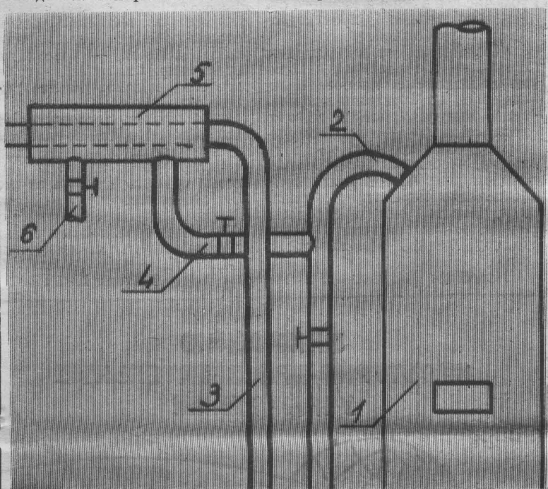
РИС. 1. СХЕМА ПАРОВОГО ПОДОГРЕВАТЕЛЯ: 1. Паровой котел. 2. Паропровод котла. 3. Водопроводная труба. 4. Паропровод, подводящий пар к подогревателю. 5. Подогреватель. 6. Устройство для сброса конденсата.
