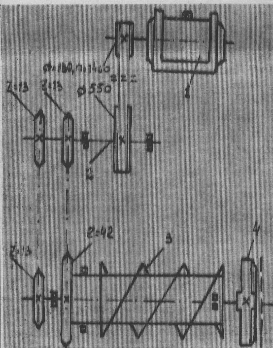
Рис. 1. Кинематическая схема пастоизготовителя ПЗГ — 2. 1—электродвигатель; 2—контрпривод; 3—шнел; 4—нож.
