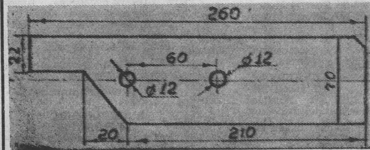
Рис. 2. Деревянный скребок для транспортера ТСН — 2А.
