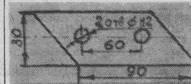
Рис. 3. Пластина для упрочнения деревянного скребка.
