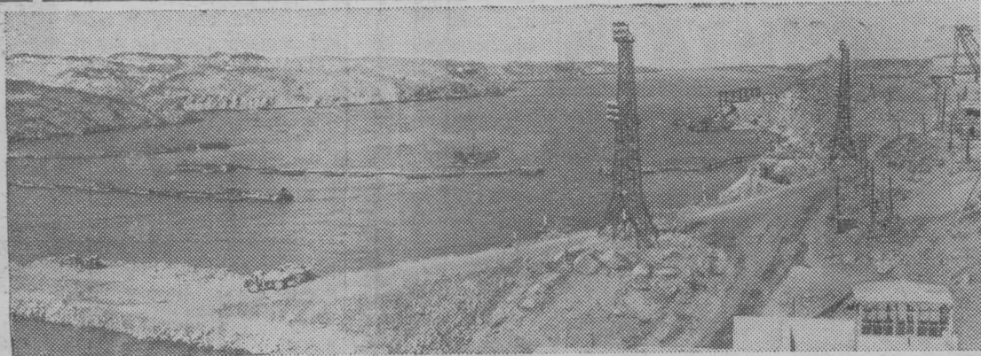
На строительстве высотной Асуанской плотины в Объединенной Арабской Республике. Перекрытие Нила состоялось 15 мая. В этот день каменно-песчаная плотина навсегда перегородила старое ложе реки. Могучий Нил понес свои воды по новому руслу—обводному каналу. Фотохроника ТАСС.
