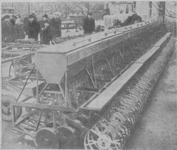
Москва. Посетители Выставки достижений народного хозяйства СССР могут увидеть среди новинок сельскохозяйственной техники широкозахватную универсальную сеялку «СП-15» с шириной захвата от 16 до 20 метров.
