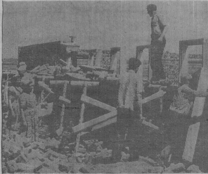
НА СНИМКЕ: плотник В. Шиталов устанавливает перекрытие свинарника-маточника на первой ферме.
