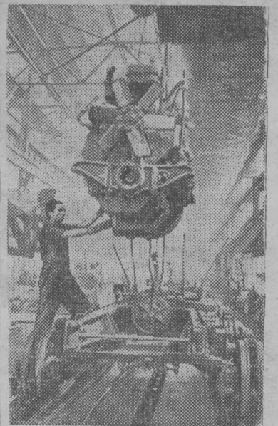
НА СНИМКЕ: главный конвейер сборки тракторов «С-100». Фото В. Соболева. Фотохроника ТАСС.
