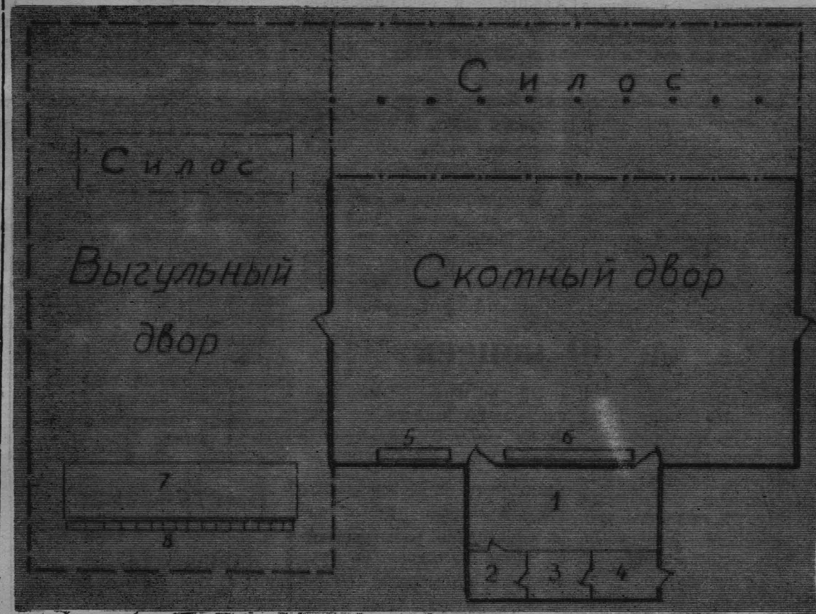
План скотного двора в совхозе «Томский» 1 — доильный зал, 2, 3, 4 — молокоприемный пункт, машинное отделение и красный уголок, 5, 6 — корыта-автопоилки, 7, 8 — ясли.
